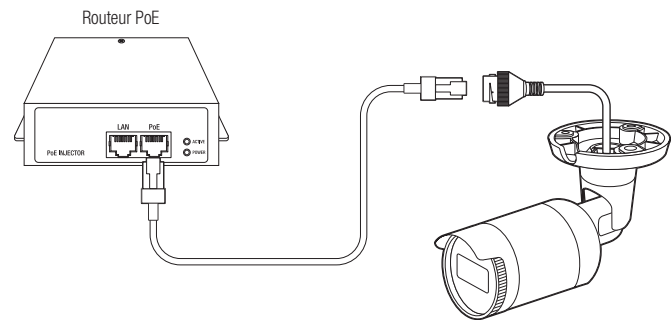
<ANO-L6082R/L7082R>
