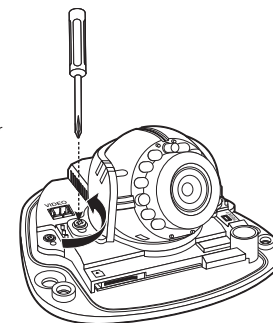
Trou de fixation
