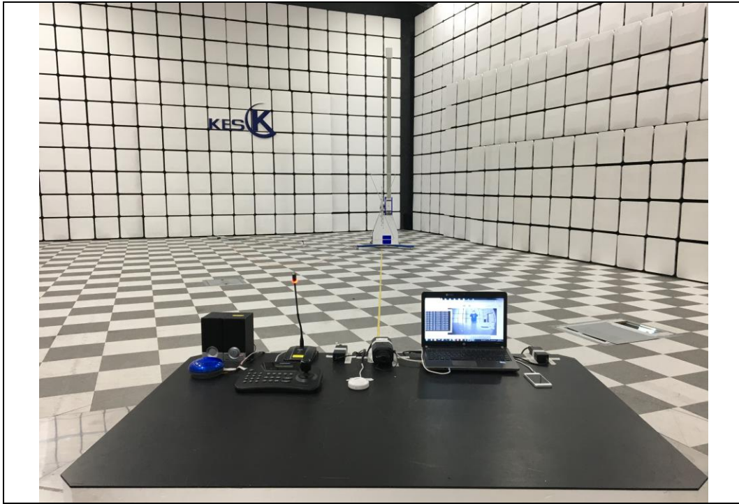
전 면 - DC 12 V Adapter 모드
