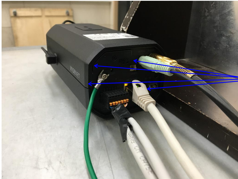
[시험기자재 - PoE Adapter 모드]
