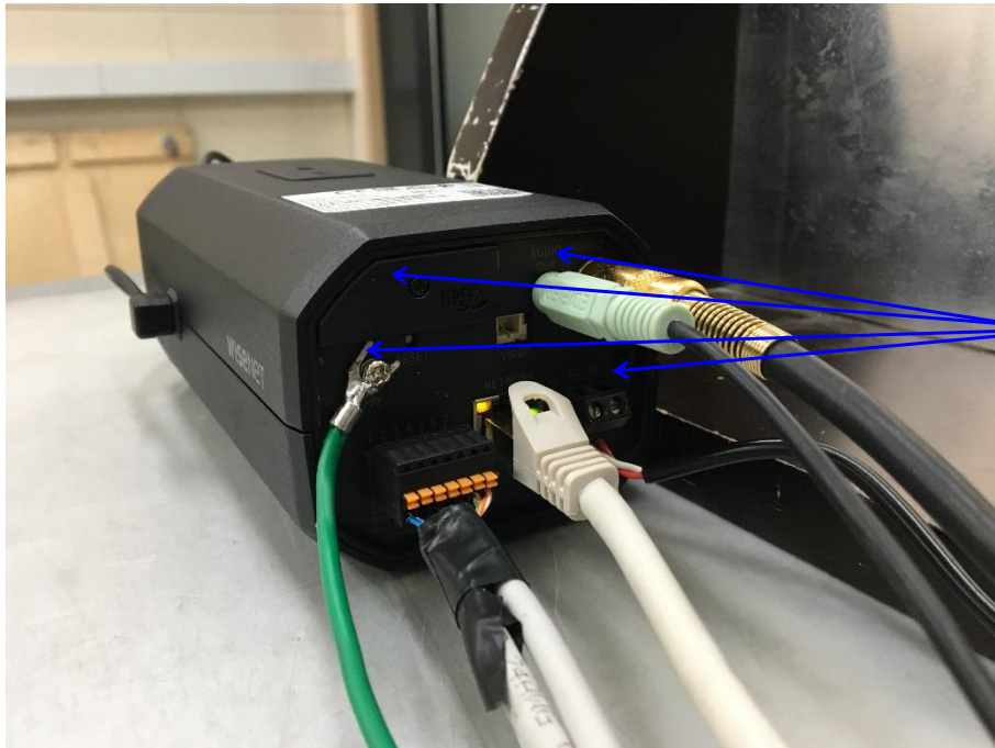
[시험기자재 - DC 12 V Adapter 모드]
