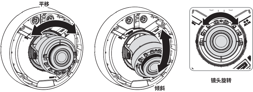
【在墙面安装时】
