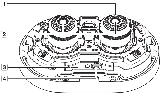
组件(前面)
