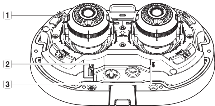
组件(背面)
