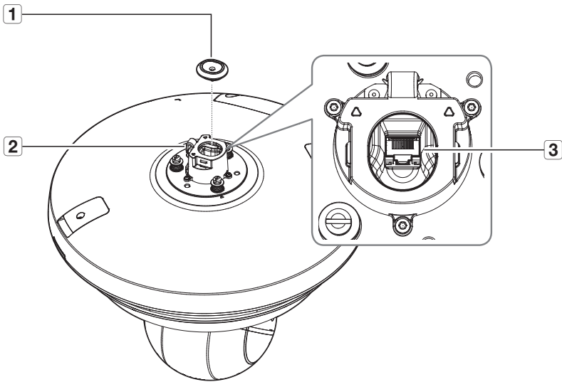
安装面
