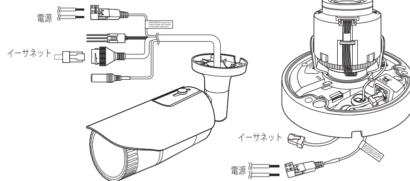
<QNO-6072R/6082R>
