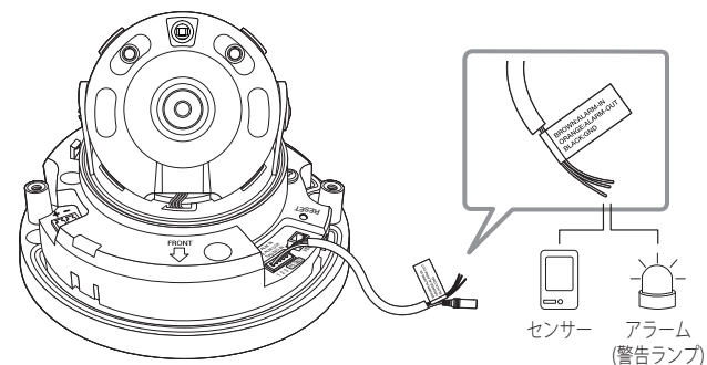
<QNV-6012R/6022R/6032R>
