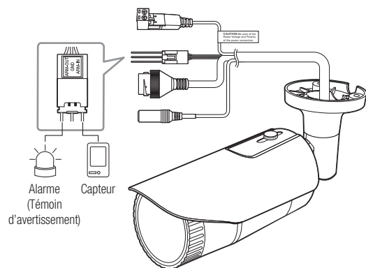
<QNO-6070R>
