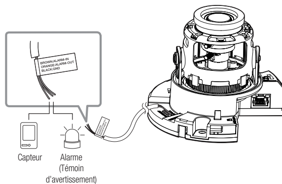
<QND-6070R>
