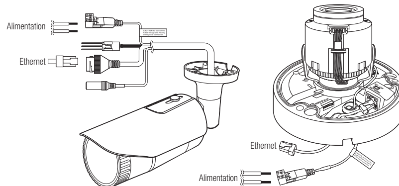
<QNO-6070R>
