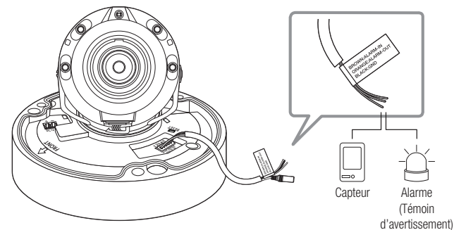
<QNV-6070R>
