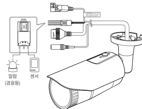
<QNV-7080R>
