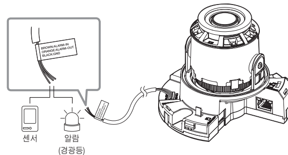
<QND-7080R>
