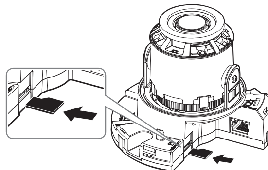
<QND-7080R>
