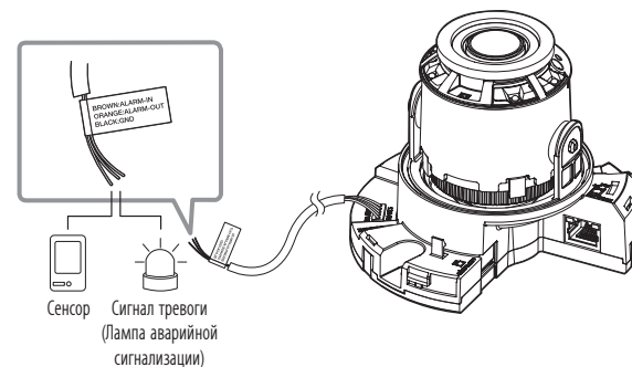
<QND-7080R>
