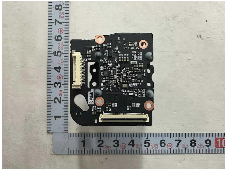
<Photo 6> IR LED 보드
