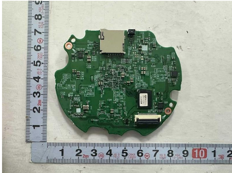
<Photo 9> 네트워크 보드
