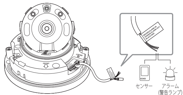
<QNV-6014R/7012R/7022R/7032R>
