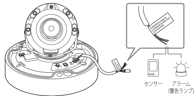
<QNV-6084R/7082R>
