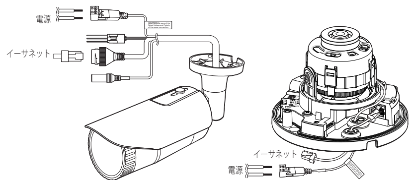
<QNO-6014R/7012R/7022R/7032R>
