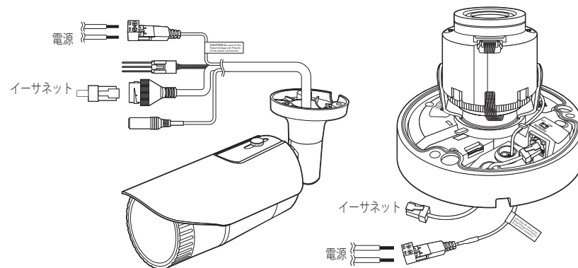
<QNO-6084R/7082R>
