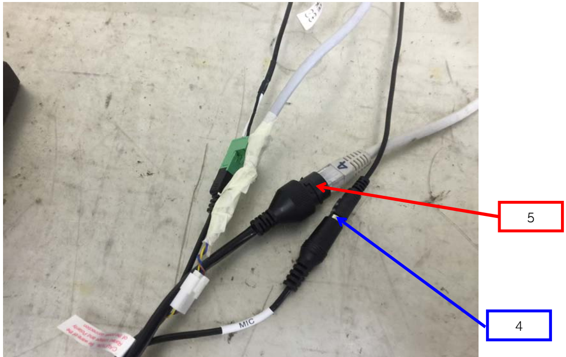
[시험기자재] - 12 V (dc), PoE 모드
