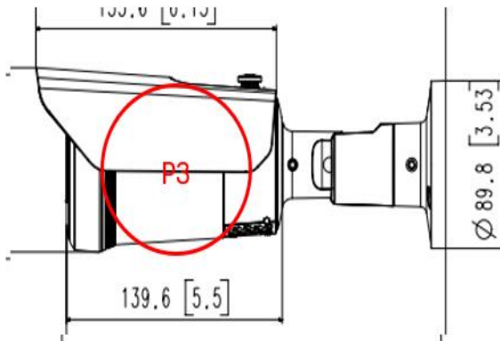
충격점 도면 표시 3
