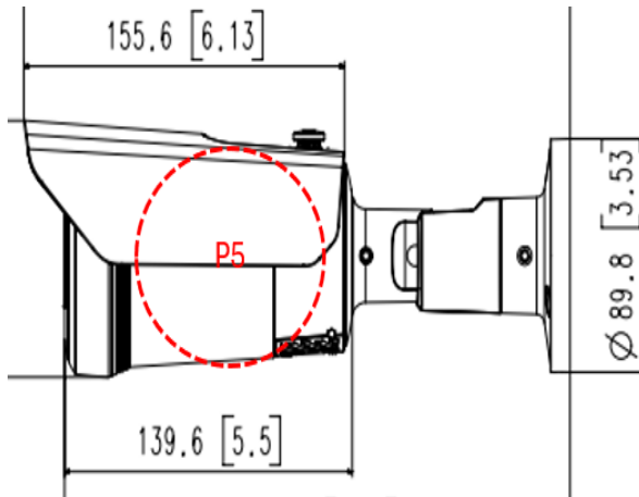
충격점 도면 표시 5
