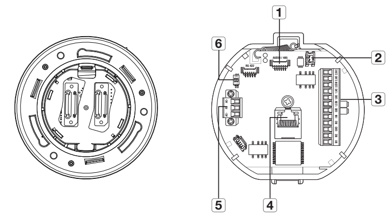
安装基座的底部视图
