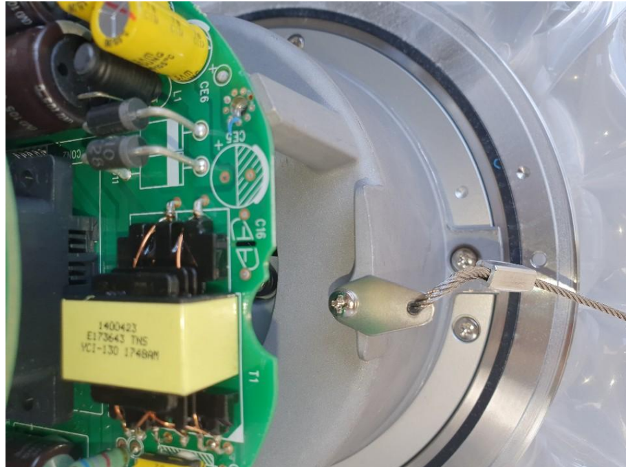
< 사진 11 > 제 1특성 숫자 시험
