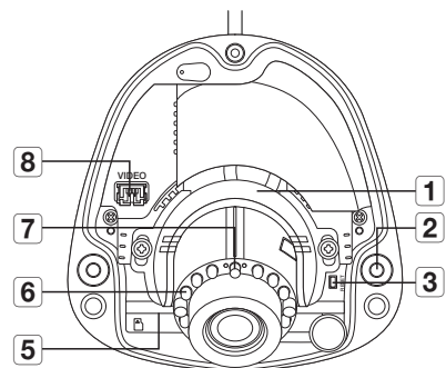
<QNV-6023R>
