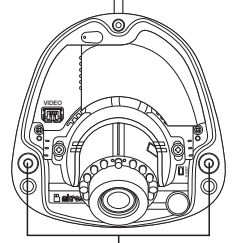
Sabitleme Deliği
