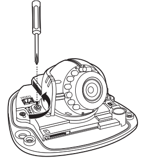
Sabitleme Deliği
