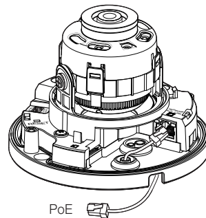
<QNV-8010R/8020R/8030R>
