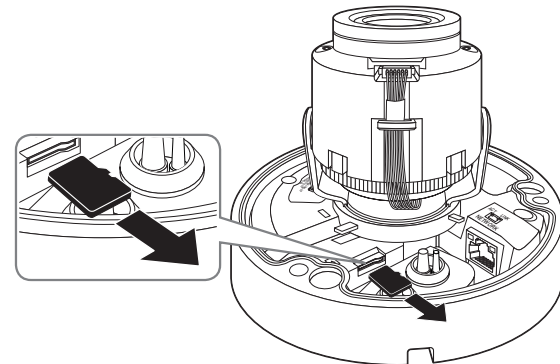
<QNV-8080R>
