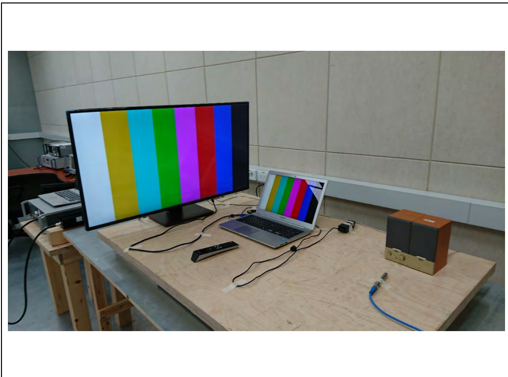
전 면-VGA 모드
