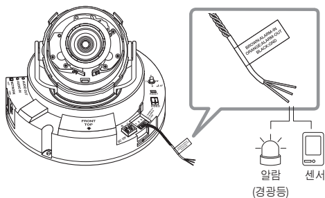
<SND-7084>
