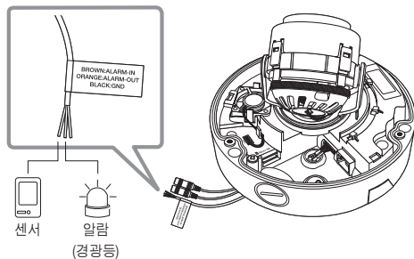
<SNV-7084>
