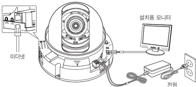
<SND-7084>
