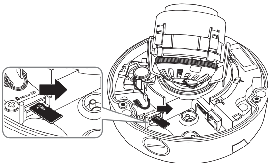
<SNV-7084>
