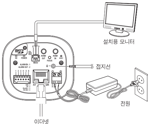
<SNB-7004>
