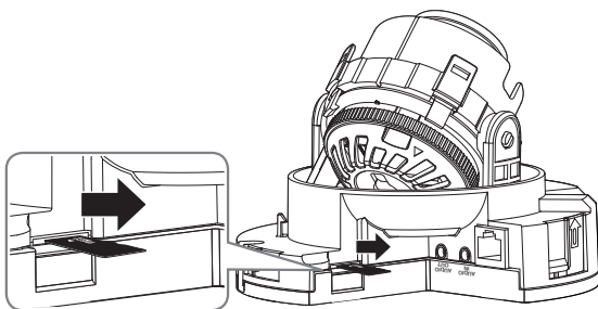
<SND-7084>
