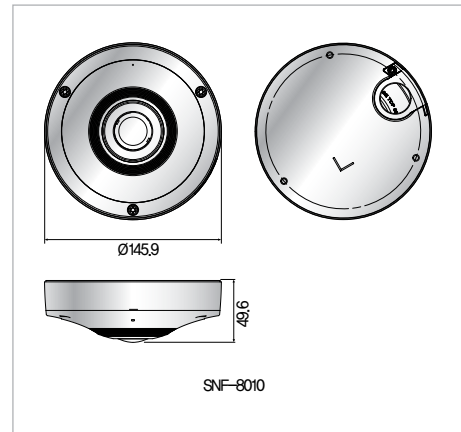
외관도
