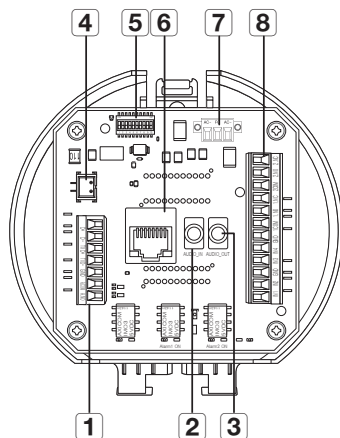
Widok podstawy instalacyjnej wewnątrz
