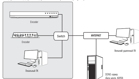
<Локальная сеть>
