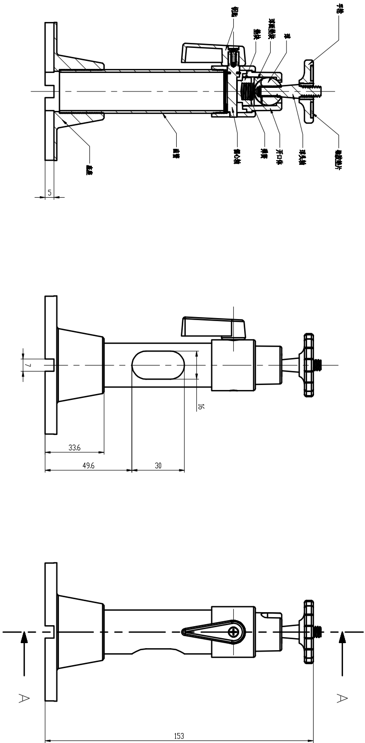
SECTION A-A
