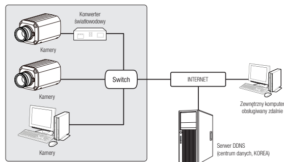
<Sieć lokalna>
