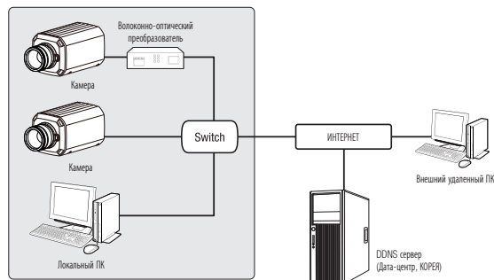
<Локальная сеть>
