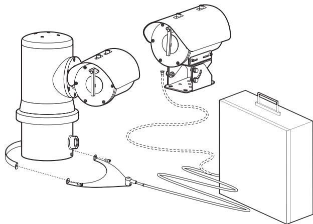
<カメラおよびウォッシャーポンプを取り付ける標準方法>
