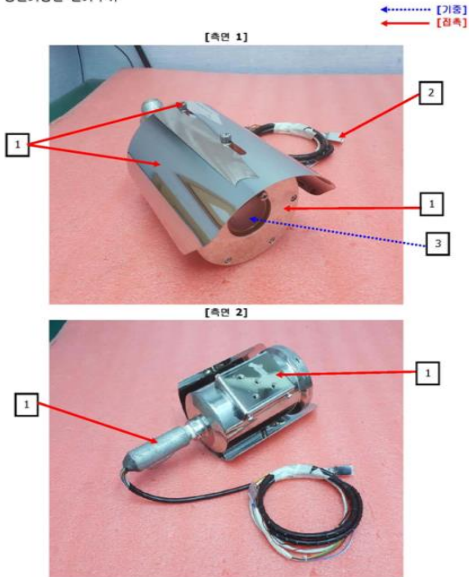
정전기방전 인가부위
