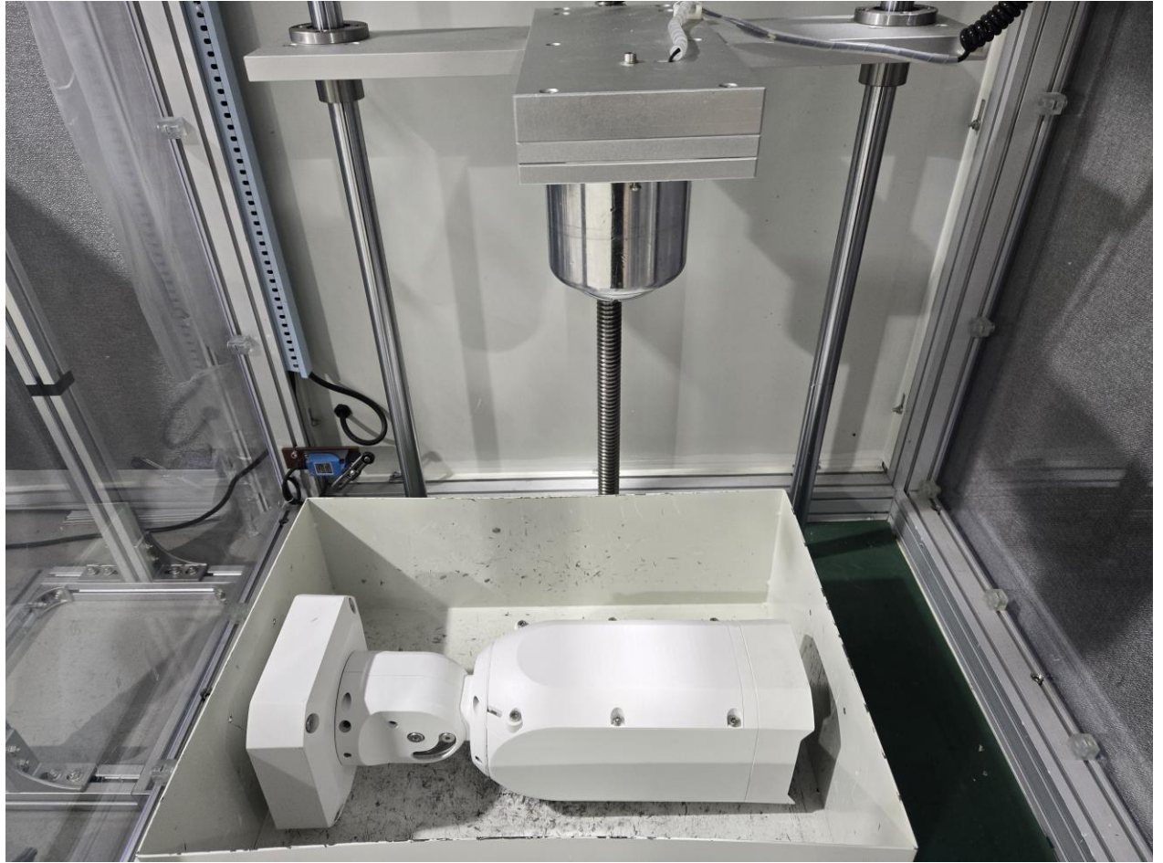
시험 환경 셋업 이미지_1
