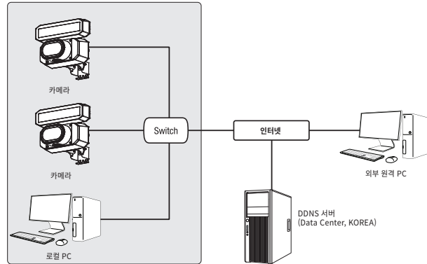
<로컬 네트워크>
