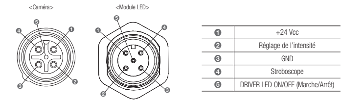
[Schéma des broches du connecteur de la caméra]
