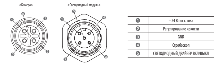
[Схема контактов разъема камеры]
