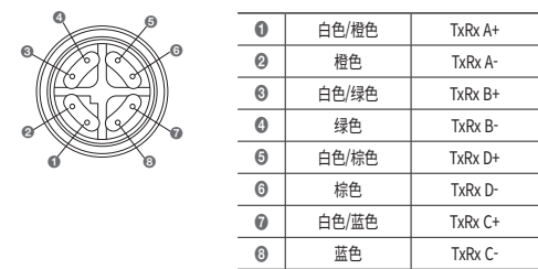
【摄像机连接器标准PIN MAP】
