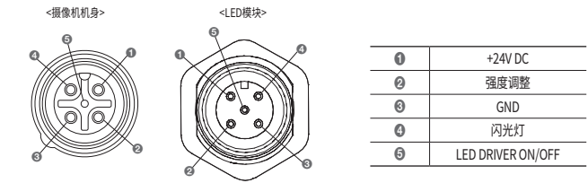
【摄像机连接器标准PIN MAP】
