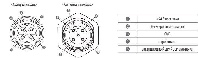
[Схема контактов разъема сканера штрихкода]
