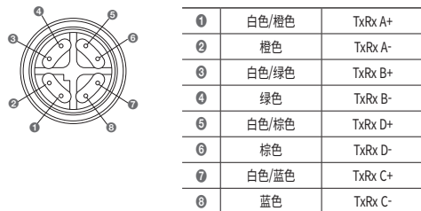
【条码扫描器连接器标准PIN MAP】
