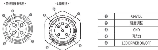
【条码扫描器连接器标准PIN MAP】
