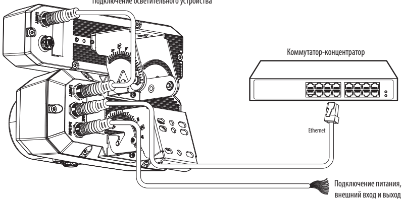
Подключение осветительного устройства
