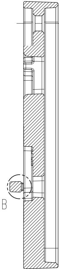
SECTION A-A
