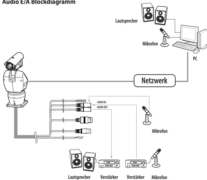
Audio E/A Blockdiagramm
