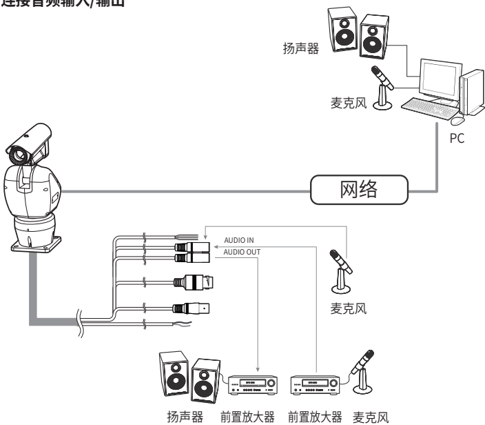
连接音频输入/输出
