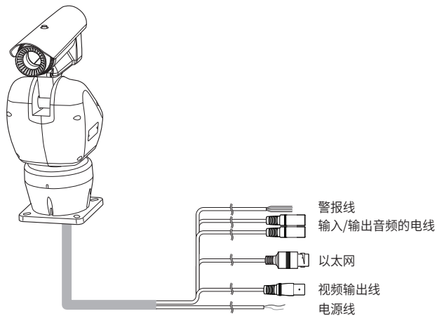
连接音频输入/输出
