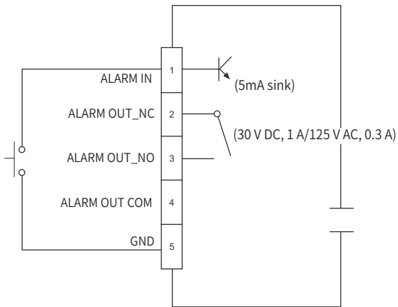
警报输入/出线线路图
