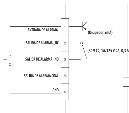
Diagrama de cableado de E/S de alarma
