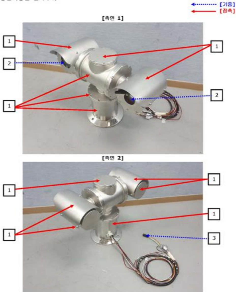
정전기방전 인가부위
