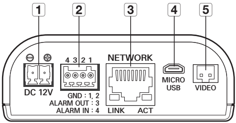
Parte trasera de la unidad principal
