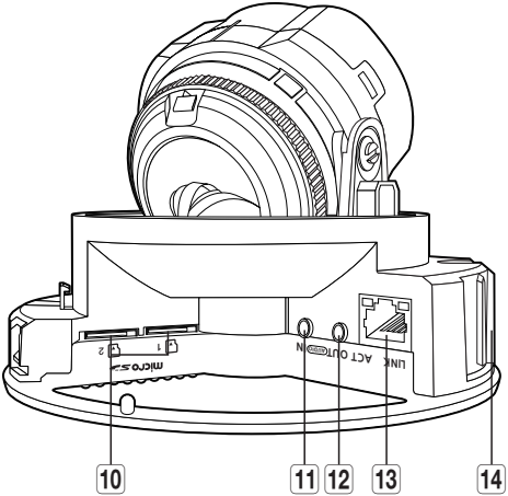
<XND-6080>
