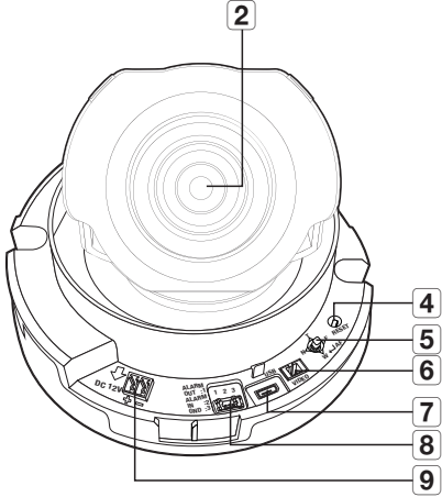
<XND-6080>
