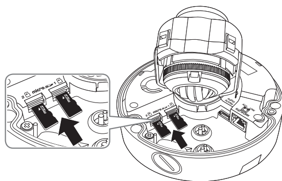
<XNV-6080/6080R/8080R>
