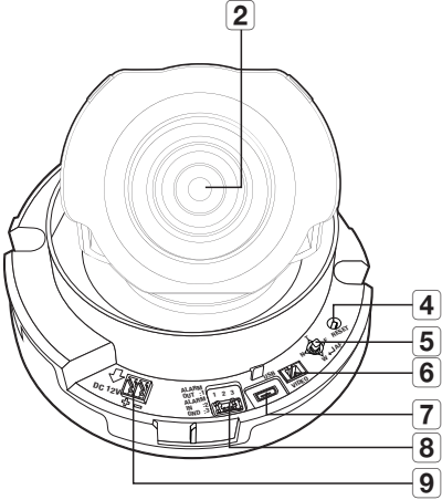
<XND-6080>
