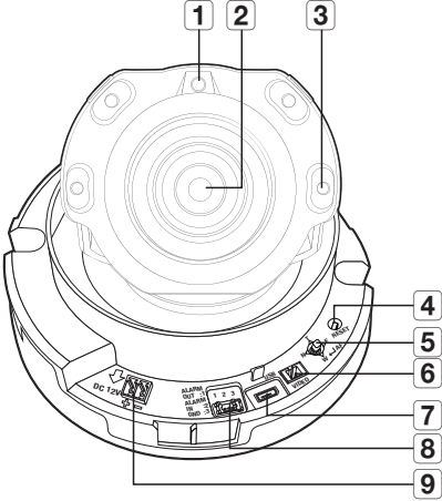
<XND-6080R/8080R>
