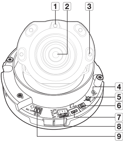
<XND-6080RV/8080RV>
