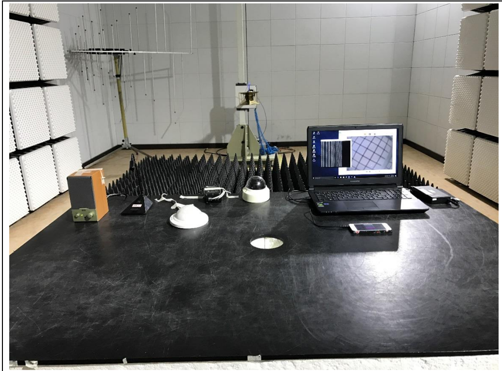
전 면 - PoE 모드
