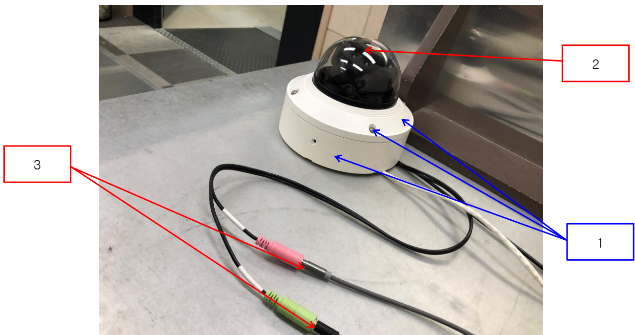
[시험기자재]_PoE 모드
