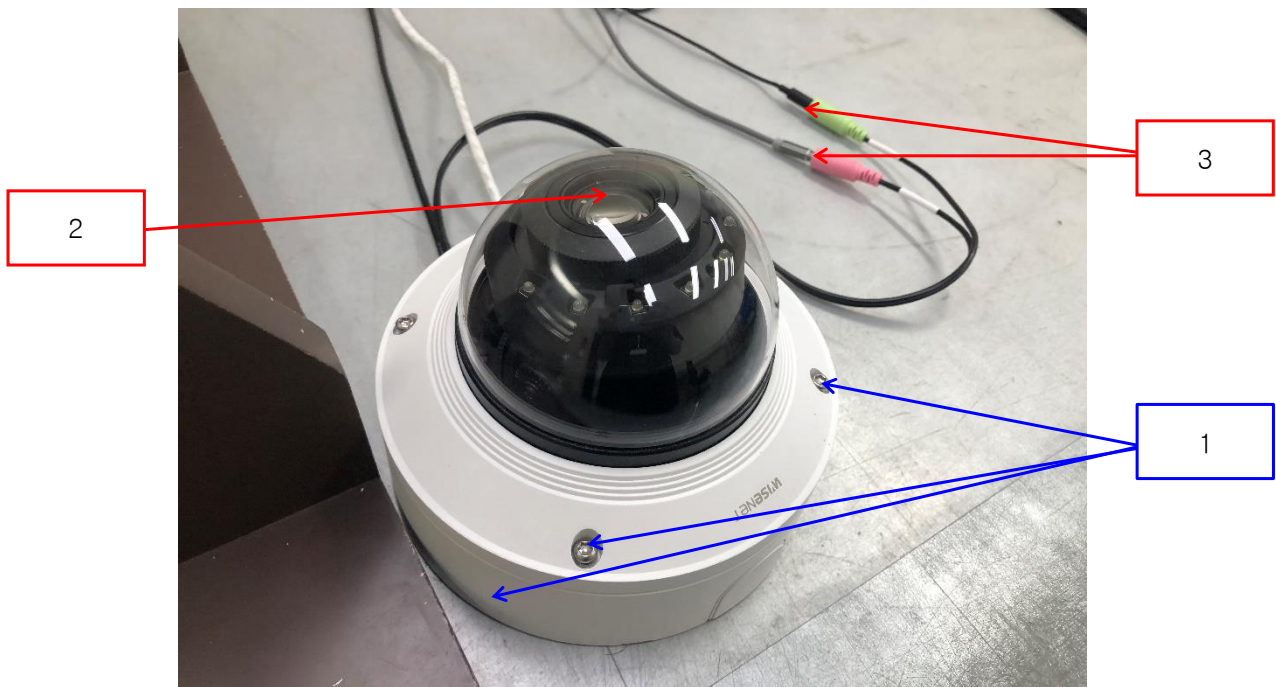
[시험기자재]_PoE 모드
