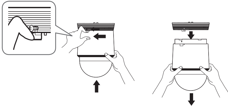
< 카메라 분리 >
