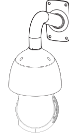
Duvara Montaj (SBP-300WM)
